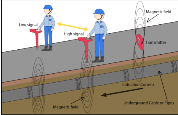
شكل (٥) - طريقة التوصيل غير المباشر
